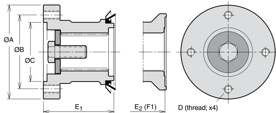
Fig. 1. DIN 90 (370 4634) (378 0642)
