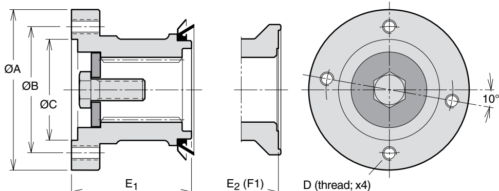
Fig. 4. SAE97 (370 4631) (378 0645)
